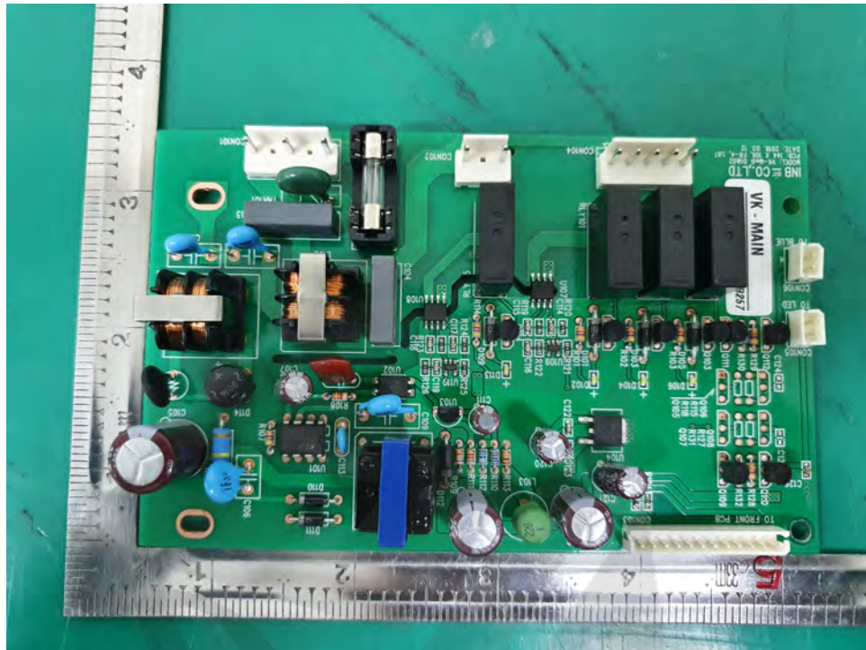
<Main PCB>
