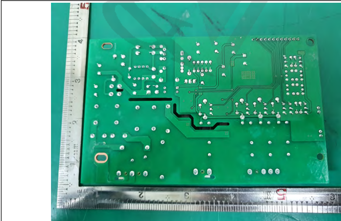
<Main PCB>
